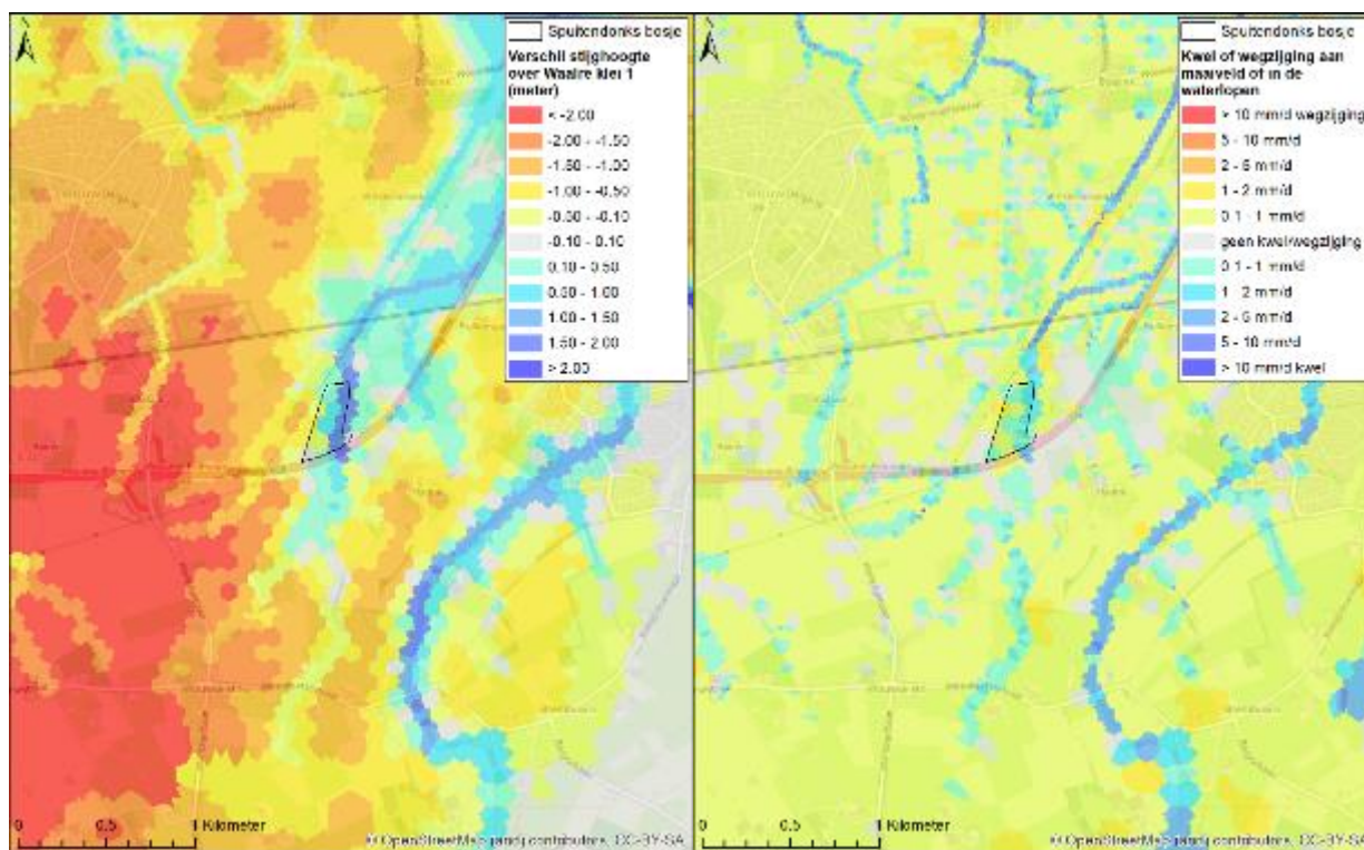
Figuur 5-5: Links: Vershill tussen stijghoogte onder de Waalre klei 1 en de grondwaterstand bij het Smitendonsbosje. Blauwe kleuren betekenen opwaartse stroming (kwel), gele en rode kleuren betekenen neerwaartse stroming (wegzijging) over deze kleilaag. Rechts: Kwel of wegzijging aan maaiveld of in de waterlopen. Blauwe kleuren geven kwel aan en geel/rode kleuren wegzijging.
