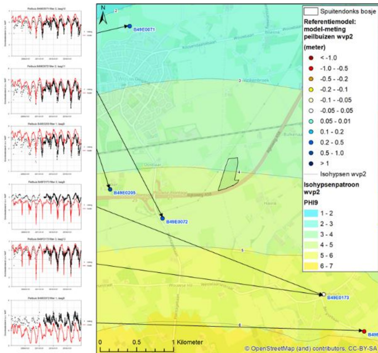
Figuur 5-3: Isohypsenpatroon in het tweede watervoerende pakket bij het Sputendons bosje. De punten tonen de locaties van de peilbuizen waarmee het model is geverifieerd. De kleur van het punt geeft aan hoeveel het model verschilt met de peilbuizen in meters. De grafieken naast de kaart tonen de verschillen tussen model en meting voor de peilbuizen in het watervoerende pakket, de rode lijn zijn gemodelleerde grondwaterstanden en de zwarte punten zijn de gemeten grondwaterstanden.
