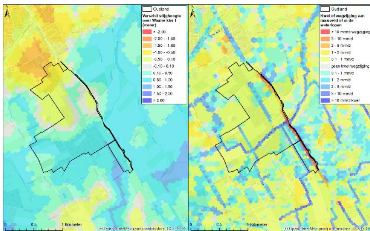
Figuur 5-3: Links: Verschil tussen stijghoogte onder de Waalre klei 1 en de grondwaterstand. Blauwe kleuren betekenen opwaartse stroming (kwel), gele en rode kleuren betekenen neerwaartse stroming (wegzijging) over deze kleilaag. Rechts: Kwel of wegzijging aan maaiveld of in de waterlopen. Blauwe kleuren geven kwel aan en geel/rode kleuren wegzijging.
