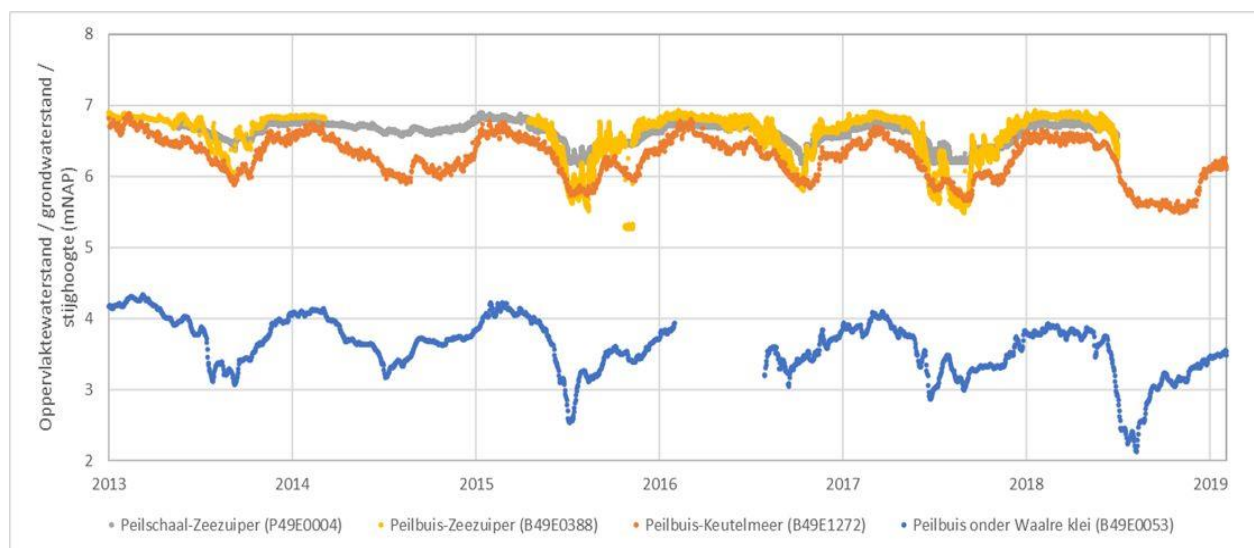
Figuur 3-20: Gemeten stijghoogte, grondwaterstand en oppervlaktewaterstand van de Zeezuiper (m+NAP). (TNO 2021; Hydronet 2021).
