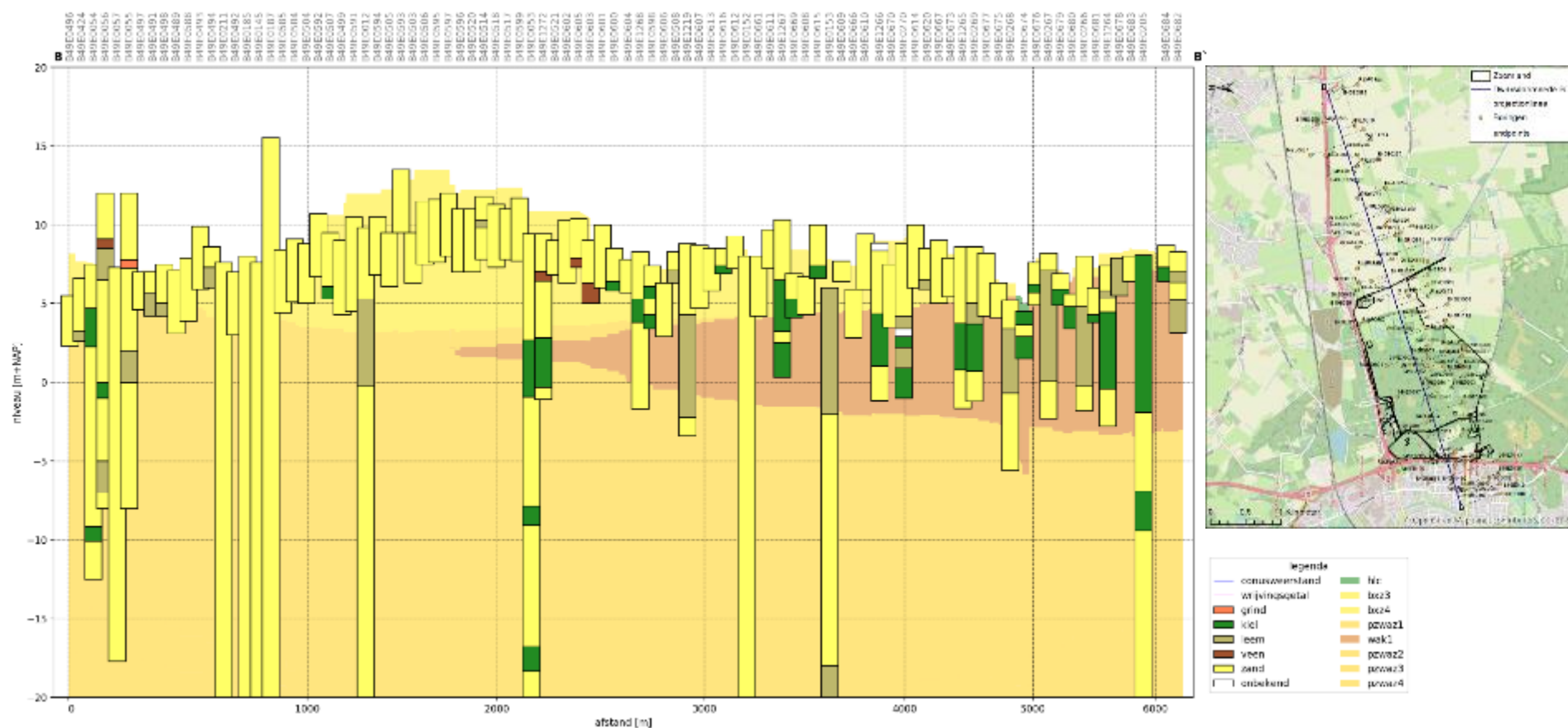
Figuur B-0-2 Geologische dwarsdoorsnede (zuid-noord) met weergave van de verschillende formaties volgens Regis II V2.2 en de beschikbare boringen (TNO 2021). Opvallend is de grote hoeveelheid boringen met een ondiepe scheidende laag (veen of klei) ter hoogte van de Zeezuiper tussen 2000 en 3000 meter.
